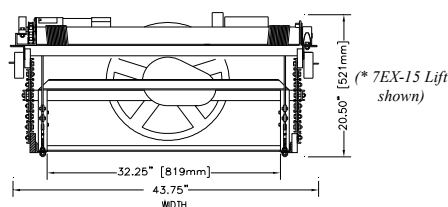
FRONT VIEW (*) (7EX-15, 7EX-18, 7EX-20, 7EX-22)
