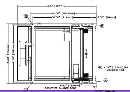
TOP VIEW (7EX-15, 7EX-18, 7EX-20, 7EX-22)
