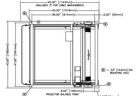
TOP VIEW (7EX-15, 7EX-18, 7EX-20, 7EX-22)
