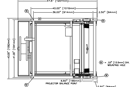
TOP VIEW (7EX-15, 7EX-18, 7EX-20, 7EX-22)
